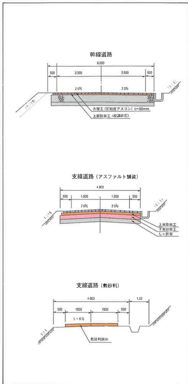
標準断面図
