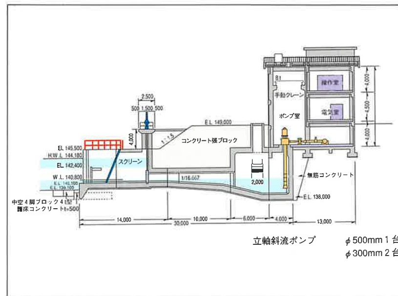
揚水機場断面図
