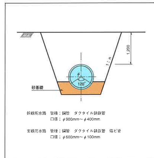
幹支線用水路標準断面図
