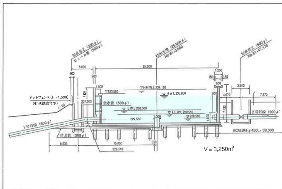
吐出水槽縦断面図
